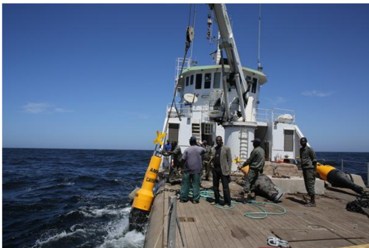
Photo 25: Opération de pose des balises dans l'AMP de Cayar par le navire Baliseur de la Direction des Phares et Balises.
